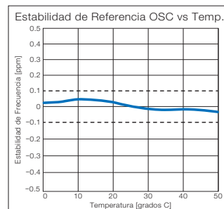
Características de deriva de temperatura TCXO ● Los valores indican ejemplos de medida.
